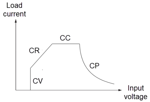
CC+CV+CP+CR mode (AUTO)
