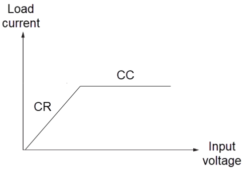
CC+CR mode
