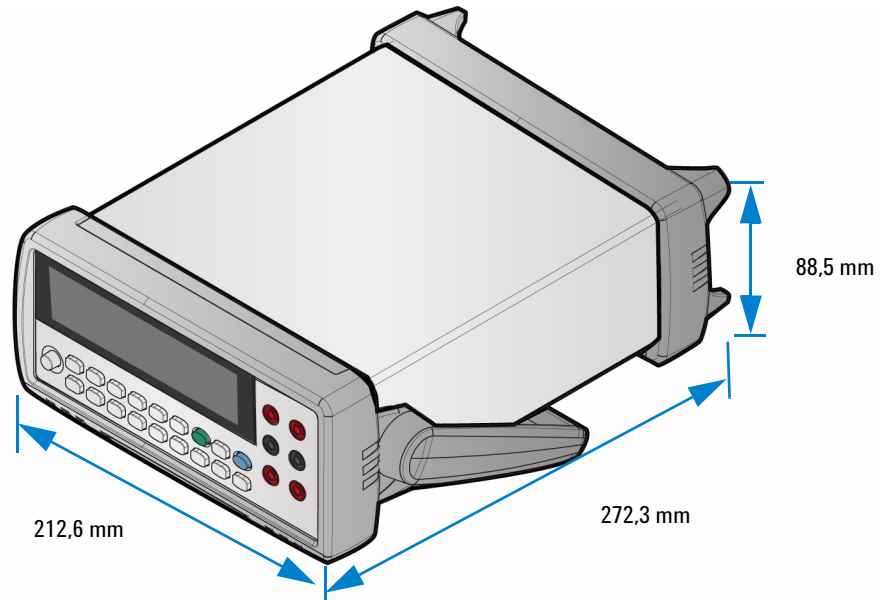
Agilent 34450A 5½ Digitales Multimeter
