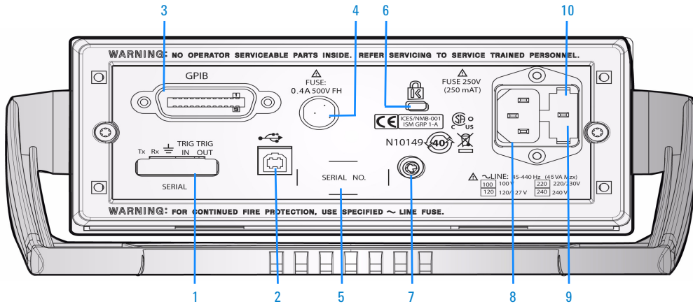
Figure 1-3 Panneau arrière d'un coup d'œil
